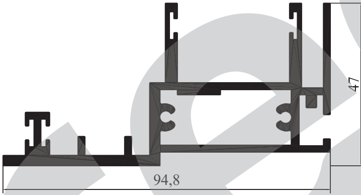
M 2372 - 2,068 kg/m
