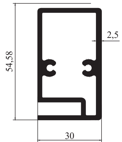
M 2371 - 1,205 kg/m
