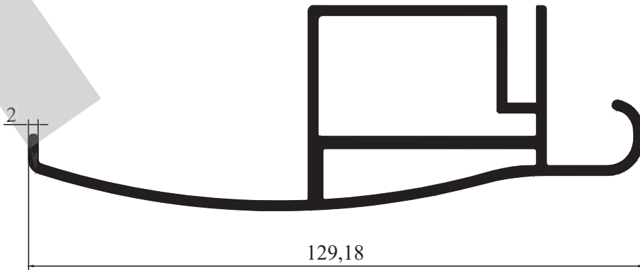
M 2373 - 1,917 kg/m
