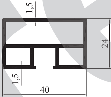
M 2055 - 0,678 kg/m
