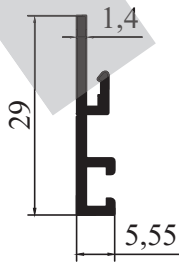
M 2052 - 0,172 kg/m
