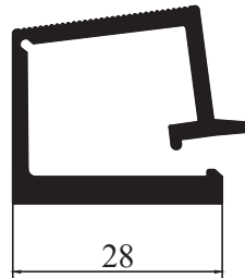
M 9561 - 0,636 kg/m
