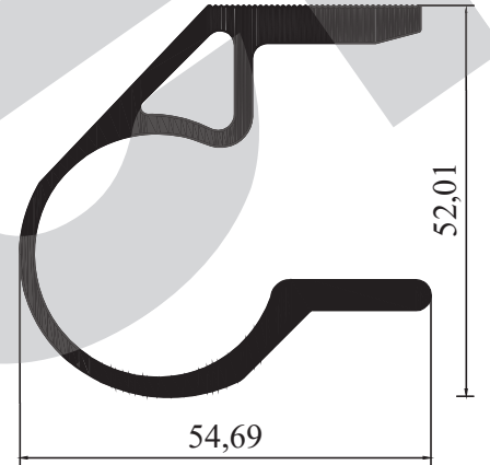
M 9562 - 1,353 kg/m
