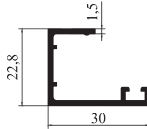
M 2050 - 0,308 kg/m
