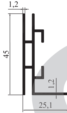
M 9202 - 0,588 kg/m
