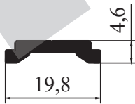
M 225 - 0,157 kg/m
