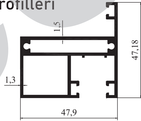
M 2054 - 0,962 kg/m
