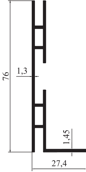
M 9521 - 0,629 kg/m
