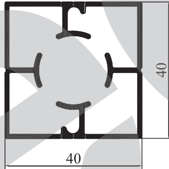
M 9540 - 0,778 kg/m
