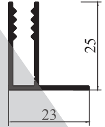
M 8502 - 0,256 kg/m
