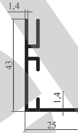
M 9201 - 0,377 kg/m
