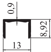
M 1500 - 0,575 kg/m
