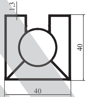
M 861 - 0,895 kg/m
