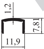
M 2011 - 0,642 kg/m
