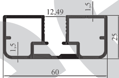
M 2073 - 0,924 kg/m
