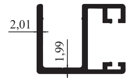
M 2057 - 0,510 kg/m
