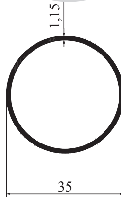
M 1528 - 0,341 kg/m
