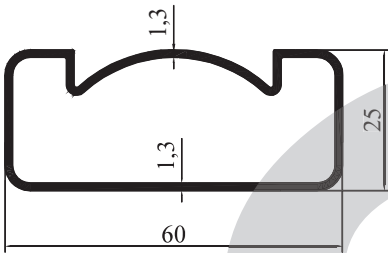
M 2078 - 0,613 kg/m
