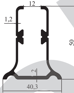
M 2064 - 0,748 kg/m
