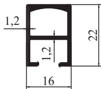
8948 - 0,265 kg/m
