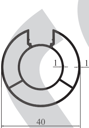
M 2011 - 0,642 kg/m
