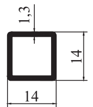
M 1416 - 0,151 kg/m
