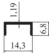
M 1528 - 0,341 kg/m
