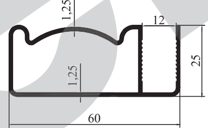
M 2075 - 0,603 kg/m
