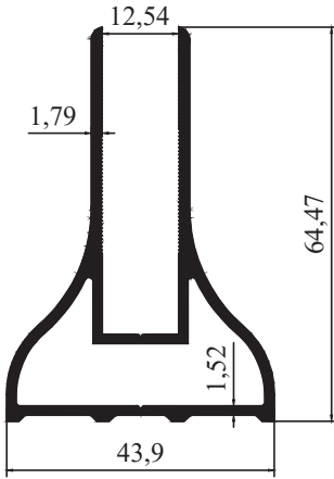
M 2061 - 0,977 kg/m
