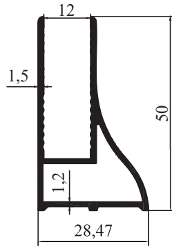
M 2062 - 0,555 kg/m
