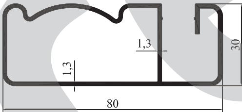
M 2076 - 0,876 kg/m
