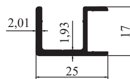
M 9532 - 0,276 kg/m
