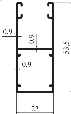
8427 - 0,420 kg/m
