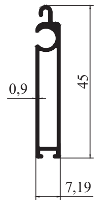
8428 - 0,277 kg/m
