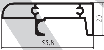
4119 - 0,544 kg/m
