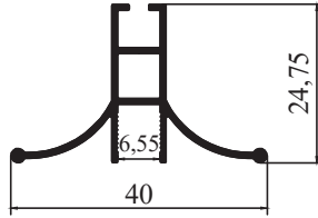
4145 - 0,284 kg/m
