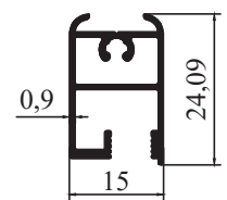
4130 - 0,254 kg/m
