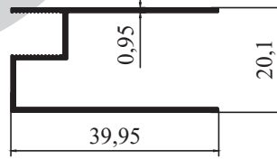
4118 - 0,273 kg/m
