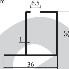
4144 - 0,289 kg/m
