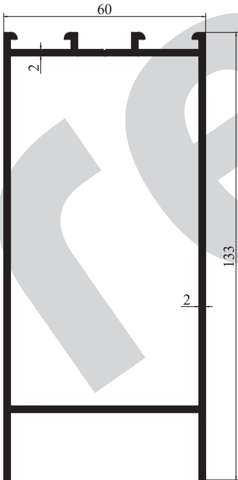
M 3109 - 2.138 kg/m
