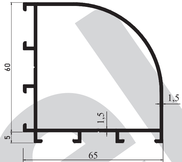
M 3106 - 1.118 kg/m
