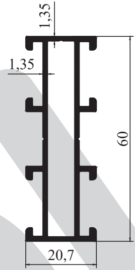
M 9515- 0,764 kg/m
