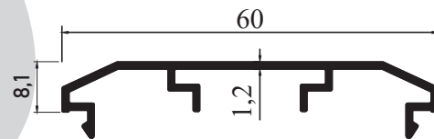
M 3108 - 0.342 kg/m
