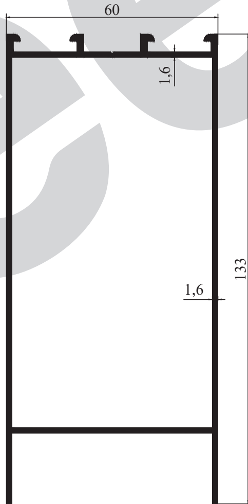
M 3104 - 1,800 kg/m
