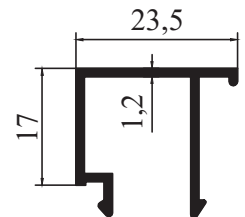
M 3111 - 0.233 kg/m
