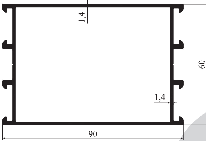
M 9514- 1,328 kg/m
