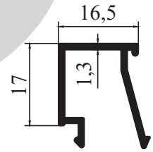
M 3112 - 0.225 kg/m
