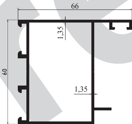
M 3105 - 1.008 kg/m
