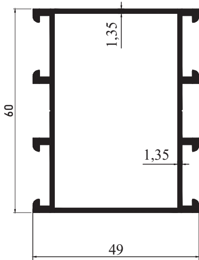
M 3101 - 0.992 kg/m
